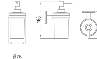
53160 DISPENSER DOSEUR ДОЗАТОР
