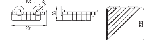
53171 CORNER WIRE RACK 20X21X8 ÉTAGÈRE D'ANGLE GRILLE 20X21X8 УГЛОВОЙ КОНТЕЙНЕР 20X21X8
