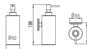
53159 DISPENSER DOSEUR ДОЗАТОР
