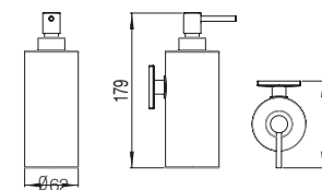
53187 DISPENSER DOSEUR ДОЗАТОР ● 00 Chrome | Chrome | Хром
