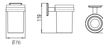
53200 BRUSH HOLDERS PORTE-COREAUX ДЕРЖАТЕЛЬ ДЛЯ ЧИПСОВ ● 00 Chrome | Chrome | Хром
