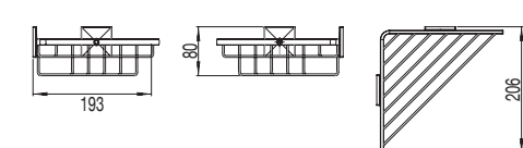
53199 CORNER WIRE RACK 20X21X8 ÉTAGÈRE D'ANGLE GRILLE 20X21X8 УГЛОВОЙ КОНТЕЙНЕР 20X21X8 ● 00 Chrome | Chrome | Хром
