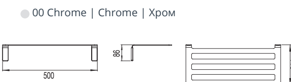
53223 TOWEL RACK ÉTAGÈRE D'HÔTE ПОЛОТЕНЦЕДЕРЖАТЕЛЬ С ПОЛКОЙ
