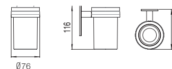
52989 BRUSH HOLDERS PORTE-COPEAUX ДЕРЖАТЕЛЬ ДЛЯ ЧИПСОВ ● 00 Chrome | Chrome | Хром ○ 01 White | Blanc | белый ● 02 Black | Noir | черный
