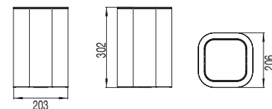
53213 WASTE BIN 5L CHROME POUBELLE 5L CHROME КОНТЕЙНЕР ДЛЯ МУСОРА 5 Л ХРОМ
