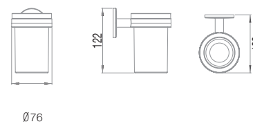
53172 BRUSH HOLDERS PORTE-COPEAUX ДЕРЖАТЕЛЬ ДЛЯ ЧИПСОВ
