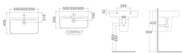
27432 SEMI-PEDESTAL With fixing kit. SEMI-COLONNE avec jeu de fixation. ПОЛУПЬЕДЕСТАЛ С установочным комплектом.
