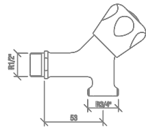
1/2" - 3/4" WASHING MACHINE TAP 48407 ROBINET LAVE-LINGE 1/2" - 3/4" КРАН ДЛЯ ПОДКЛЮЧЕНИЯ СТИРАЛЬНОЙ МАШИНЫ 1/2" - 3/4"
