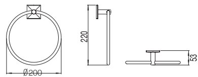
53208 TOWEL RING ANNEAU PORTE-SERVIETTES КОЛЬЦЕВОЙ ПОЛОТЕНЦЕДЕРЖАТЕЛЬ
