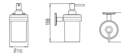
53188 GLASS DISPENSER DOSEUR ДОЗАТОР ● 00 Chrome | Chrome | Хром
