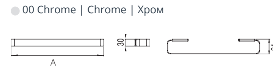
53222 TOWEL RAIL 60 CM PORTE-SERVIETTES 60 CM ПОЛОТЕНЦЕДЕРЖАТЕЛЬ 60 CM
