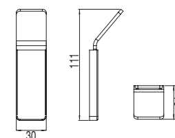
53215 ROBE HOOK PATÈRE ВЕШАЛКА ● 00 Chrome | Chrome | Хром
