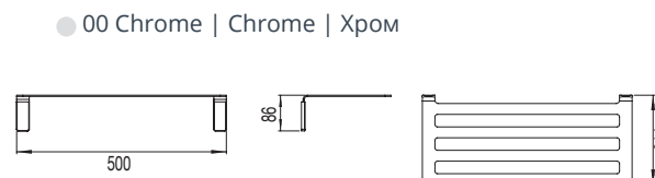
53223 TOWEL RACK ÉTAGÈRE D'HÔTE ПОЛОТЕНЦЕДЕРЖАТЕЛЬ С ПОЛКОЙ
