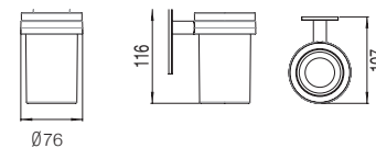
52989 BRUSH HOLDERS PORTE-COPEAUX ДЕРЖАТЕЛЬ ДЛЯ ЧИПСОВ ● 00 Chrome | Chrome | Хром ○ 01 White | Blanc | белый ● 02 Black | Noir | черный
