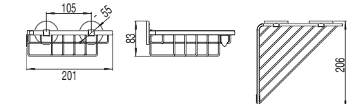
53171 CORNER WIRE RACK 20X21X8 ÉTAGÈRE D'ANGLE GRILLE 20X21X8 УГЛОВОЙ КОНТЕЙНЕР 20X21X8
