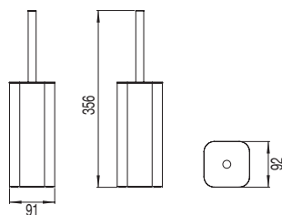
53212 FREE STANDING TOILET BRUSH BROSSE À TOILETTES À POSER НАПОЛЬНЫЙ ЕРШИК ДЛЯ УНИТАЗА ● 00 Chrome | Chrome | Хром
